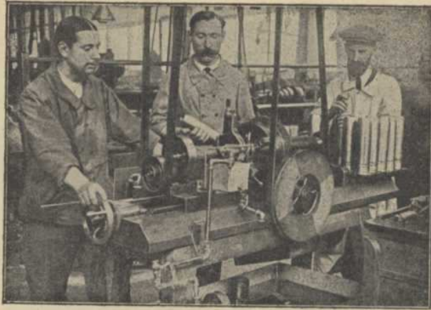
FABRICATION D'OBUS — TOURNAGE DE LA CEINTURE
